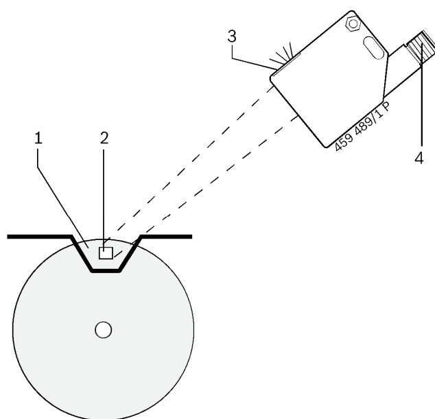
Fig.1: Optische toerentalsensor
